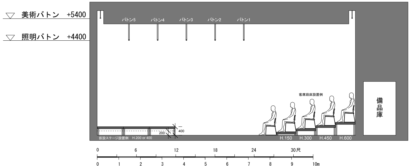
断面 B
