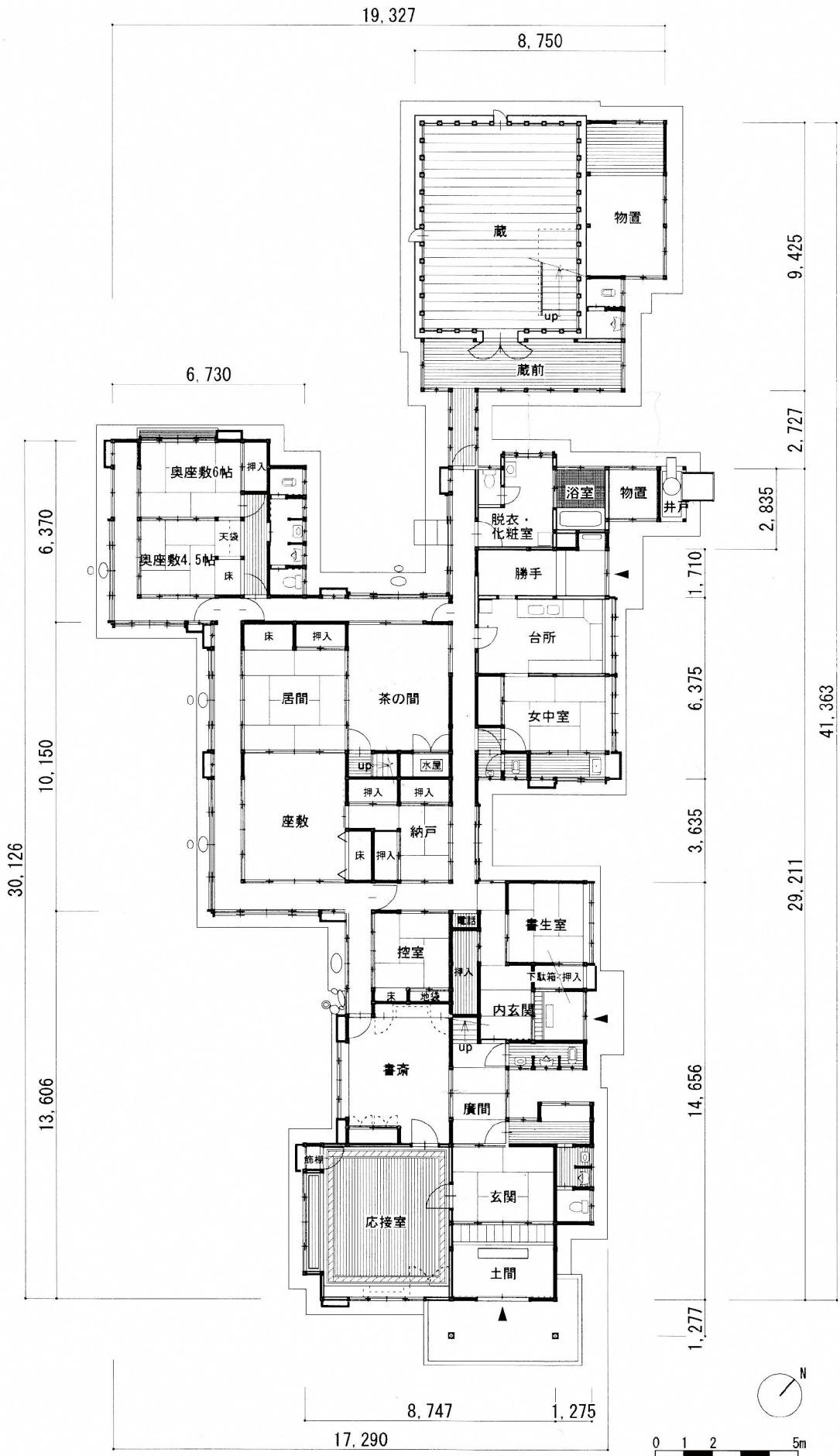
旧日本銀行新潟支店長役宅一階平面図 (縮尺 1:200)
